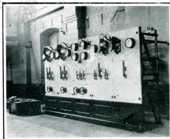
"Switch board" ó tablero de distribución
